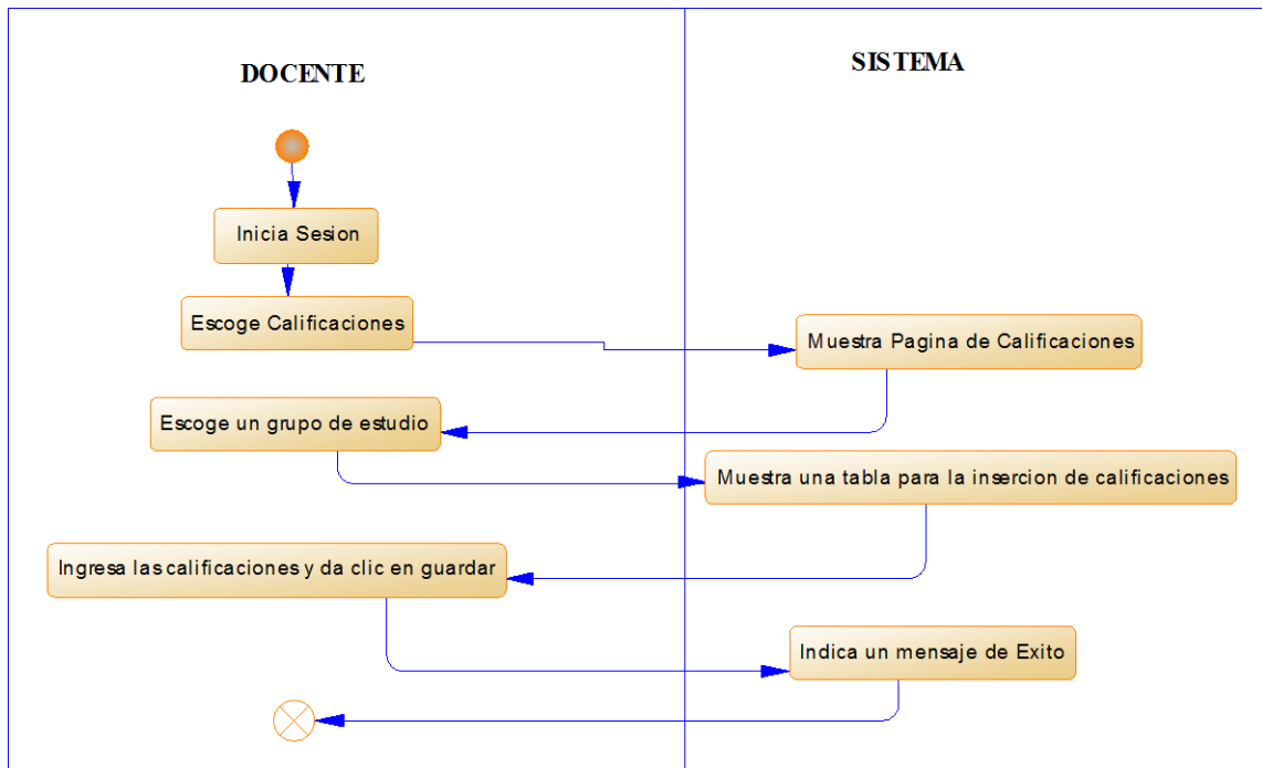
Figura 89: Diagrama de Actividad Ingresar otras Calificaciones
