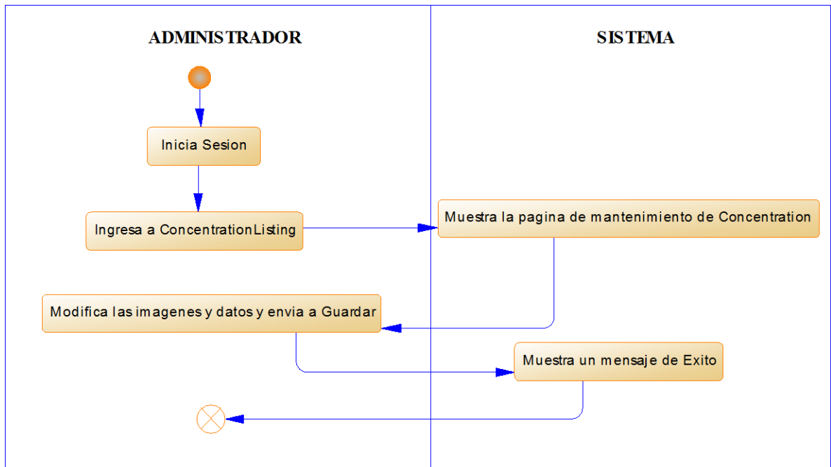
Figura 93: Diagrama de Actividad Modificar Concentration
