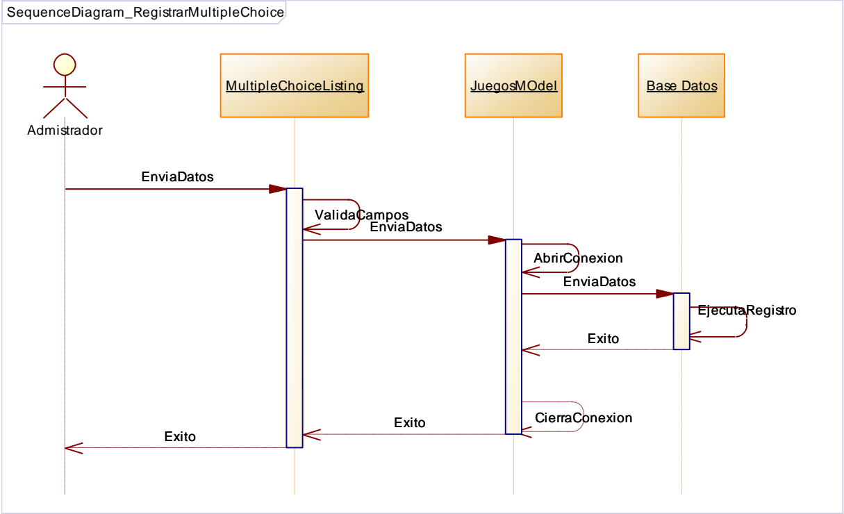
Figura 65: Diagrama de Secuencia Registrar Multiple Choice
