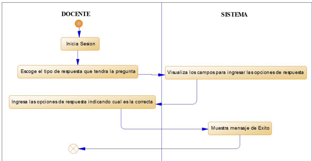
Figura 84: Diagrama de Actividad Registrar Opciones de Respuesta
