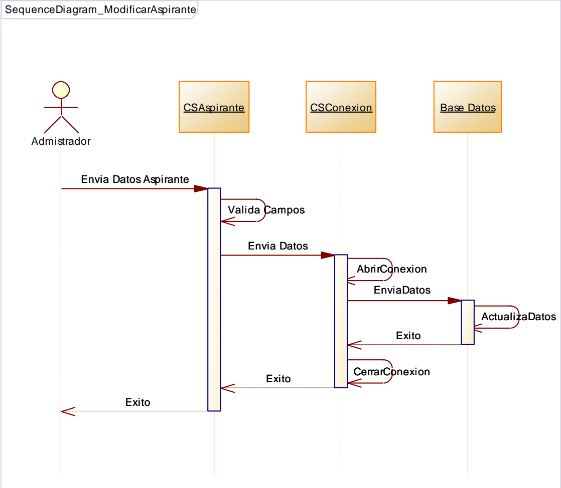
Figura 43: Diagrama de Secuencia Modificar Aspirante
