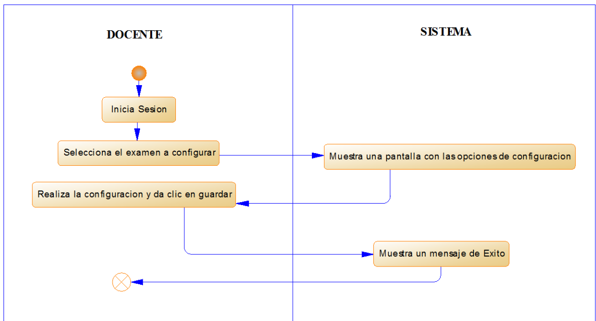
Figura 85: Diagrama de Actividad Configurar Exámenes
