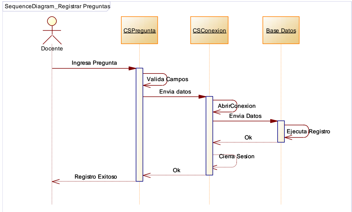
Figura 53: Diagrama de Secuencia Registrar Pregunta
