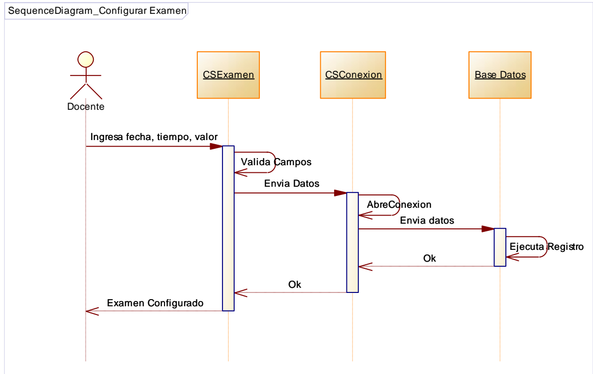
Figura 55: Diagrama de Secuencia Configurar Exámenes
