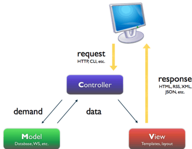
Figura 3: Arquitectura Modelo-Vista-Controlador
