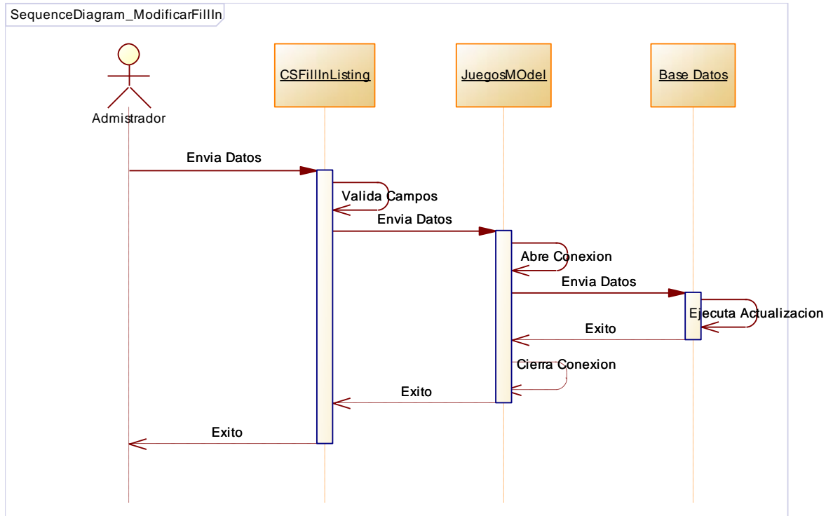
Figura 69: Diagrama de Secuencia Modificar Fill In
