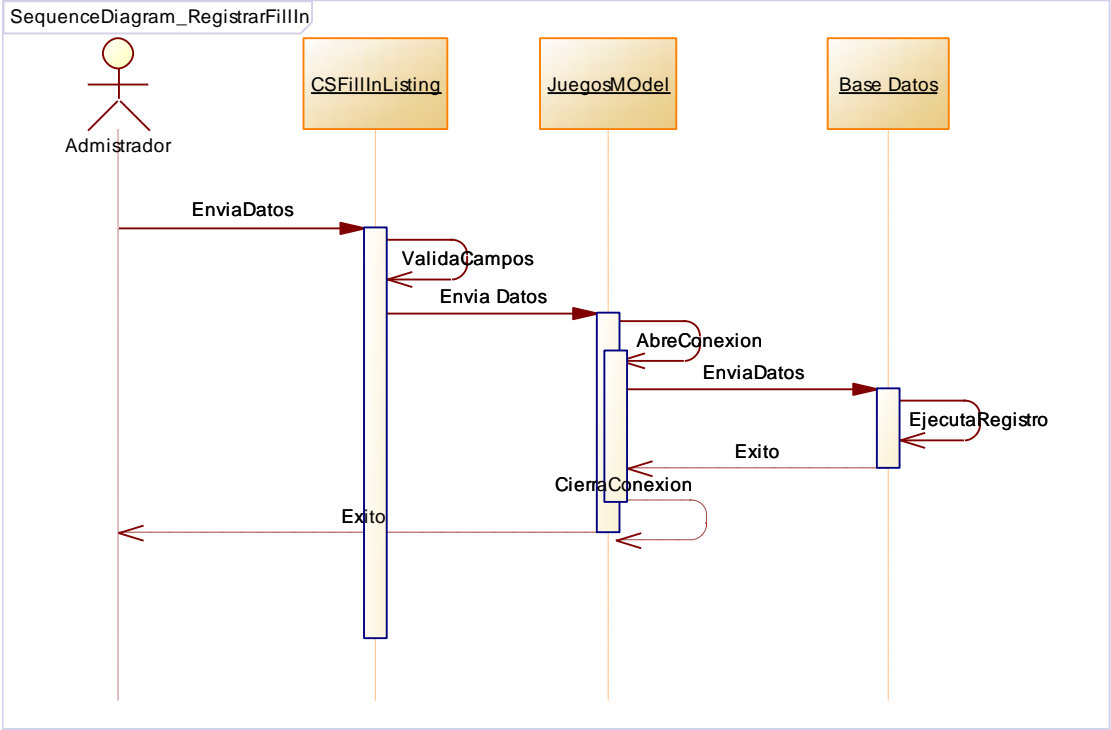
Figura 68: Diagrama de Secuencia Registrar Fill In
