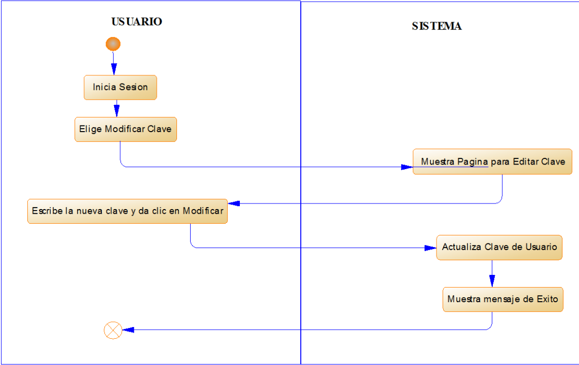
Figura 77: Diagrama de Actividad Cambiar Contraseña
